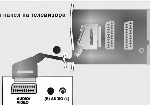
Видеокасетофон
