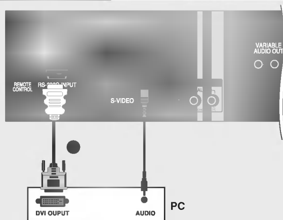
Заден панел на телевизора
