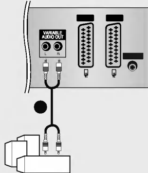
Аналогов стереоусилвател
