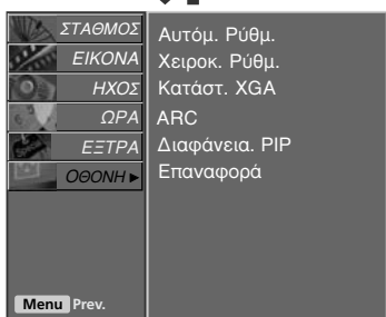
Μενού ΟΘΟΝΗ
