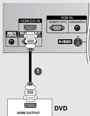
Заден панел на телевизора
