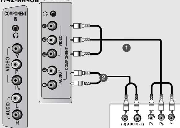
Ресивър за DTV (цифрова телевизия) (сет-топ-бокс)
