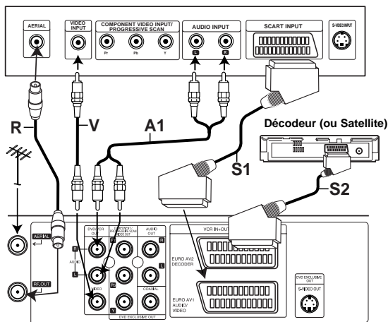
L'arrière de l'appareil (Branchement de base)
