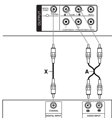
Усилитель (ресивер)
