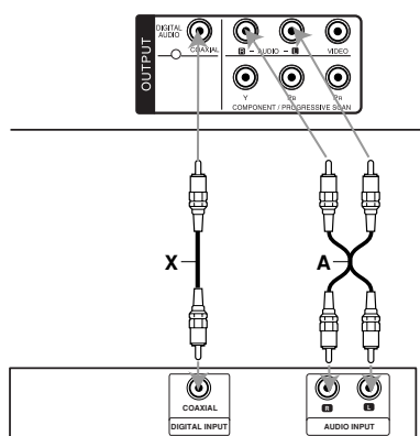
Усилитель (ресивер)
