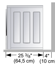
[Vue latérale]
