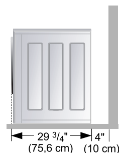
[Vue latérale]
