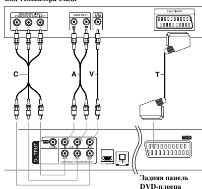
Вид телевизора сзади
