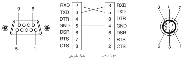
<الشكل ١، كابل واجهة RS-232C>
