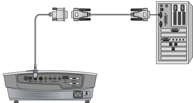
<الشكل ١، كابل واجهة RS-232C>
