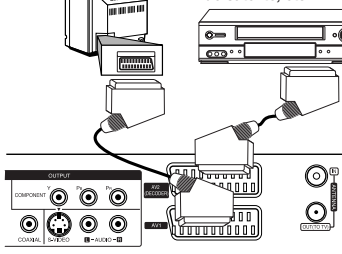
Panel posterior de la grabadora
