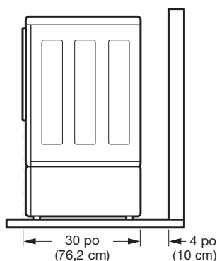
Dimensions requises pour installation avec piédestal
