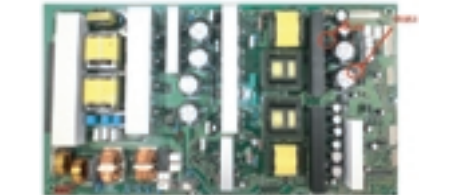
(Illustrazione.3) Tensione Del Assy del PWB Di Alimentazione Di 60inch FHD.
