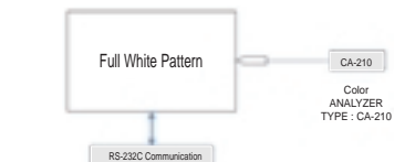
(Illustrazione. 3) Diagramma di collegamento della regolazione automatica W/B.
