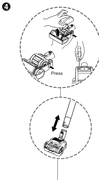
④ Mini turbine nozzle (optional)
