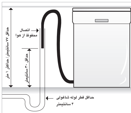
شکل ب : اتصال تخلیه - لوله شاغولی
