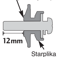
Aparāta montāžas sāns (ar starpliku)
