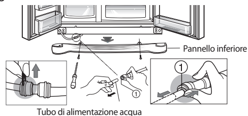
Tubo di alimentazione acqua
