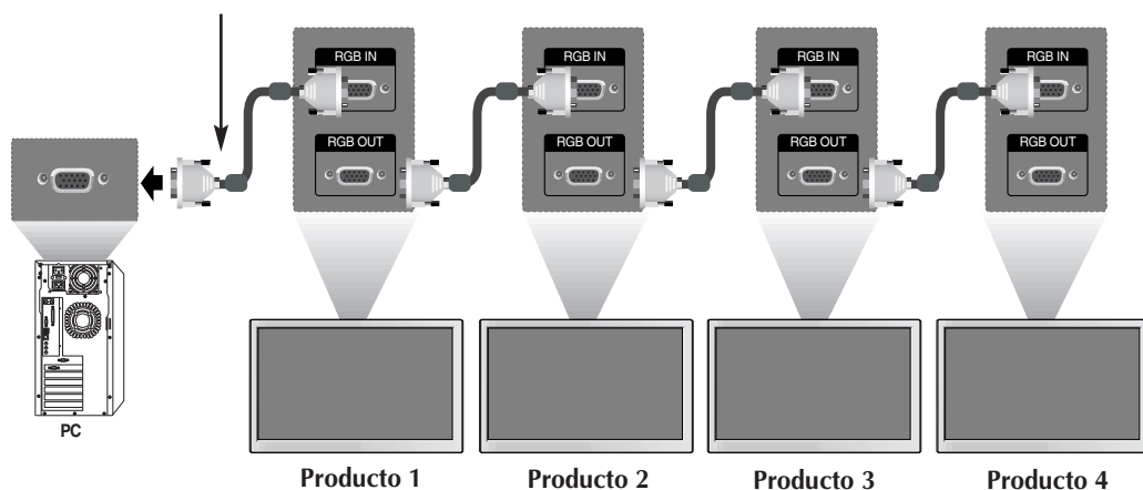
Cable de señal D-Sub de 15 patillas
