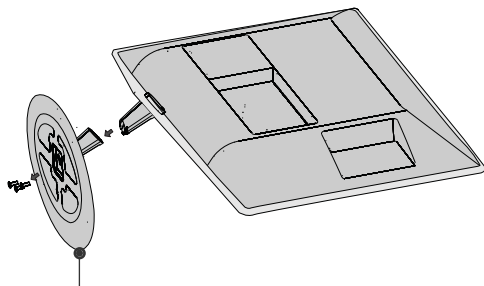
Base copertura
