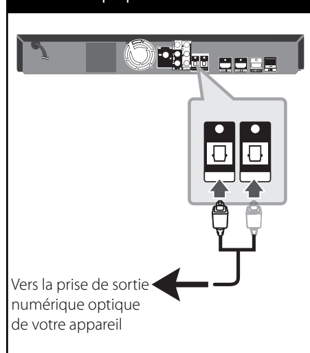
Connexion optique
