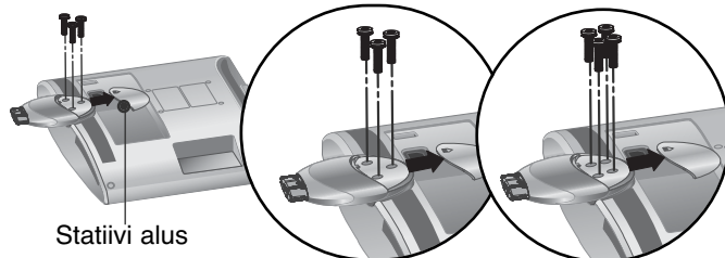
Tagumine statiiv
