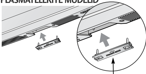
Kaitsekate
