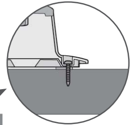
1-гвинт (постачаються як деталі продукту)
