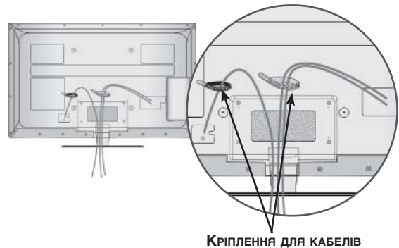
Кріплення для кабелів
