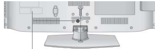
1-гвинт (постачаються як деталі продукту)
