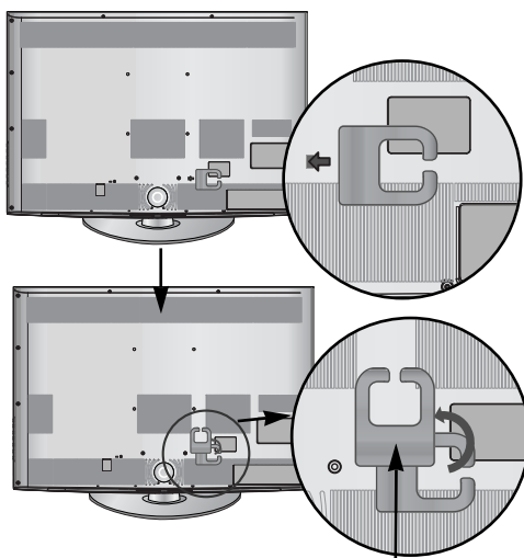
Κλιπ διαχείρισης καλωδίων
