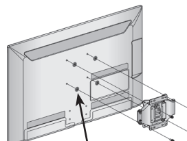
טבעות מרווח 4
