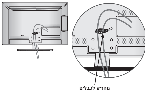
מחזיק לכבלים
