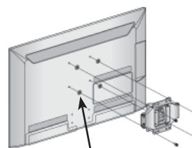
4 vaherõngast
