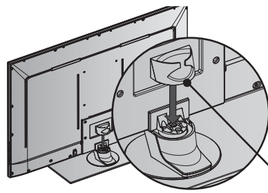
Халка за придържане на кабели
