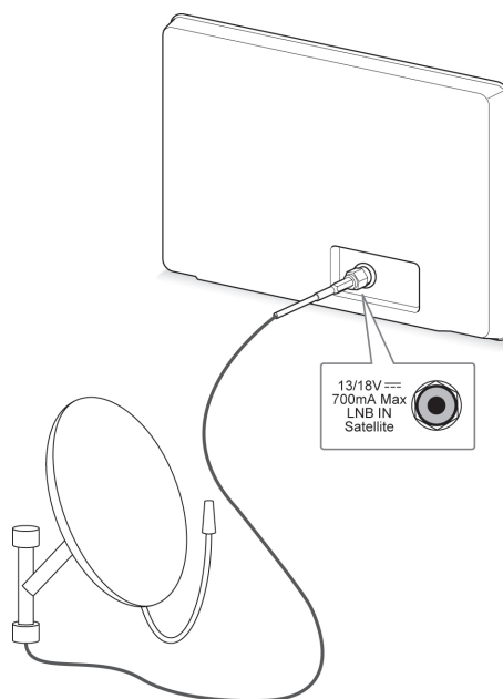
Супутникова антена
