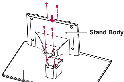
Stand Base
