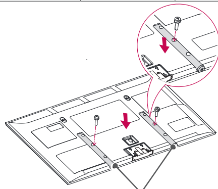
Οδηγοί στήριξης
