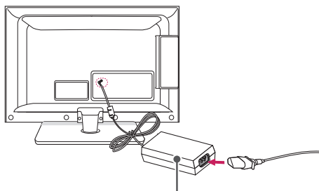
Adaptateur AC/DC
