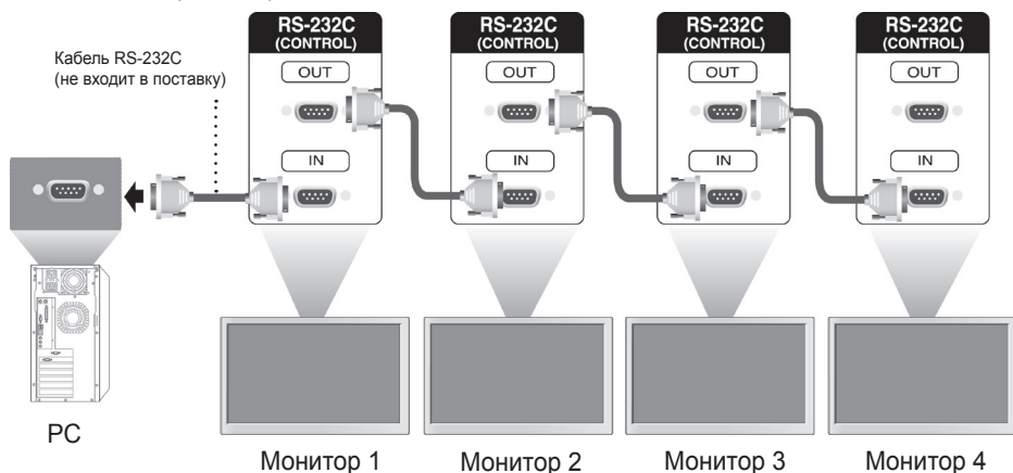
3-проводные конфигурации (нестандартный кабель)
