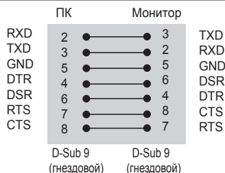
Конфигурации с 7 проводами (стандартный кабель RS-232C)
