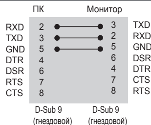
3-проводные конфигурации (нестандартный кабель)
