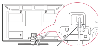
Držač Kabla za napajanje
