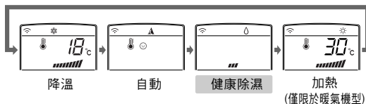
功能選擇
