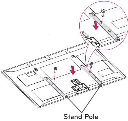
Stand Pole
