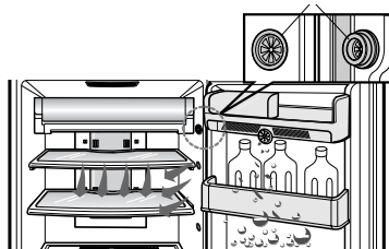
Αεραγωγός ψύξης
