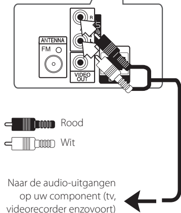
Achterkant van het apparaat
