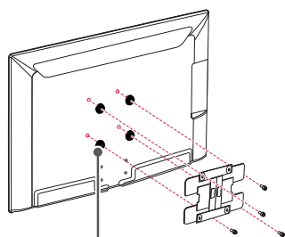
Separador interno
