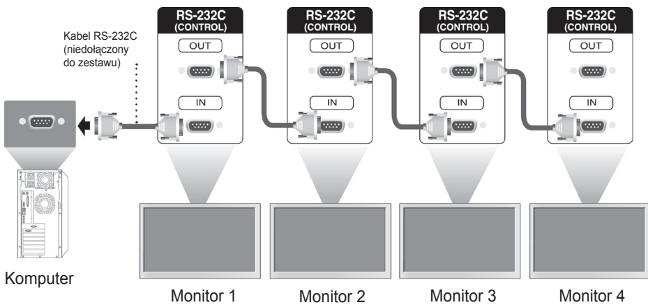
Konfiguracja 7-przewodowa (standardowy kabel RS-232C)
