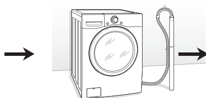
Raccordement de la conduite d'évacuation
