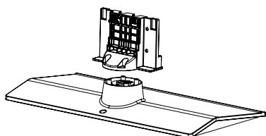
底座支架 / 底座 (仅 32/37/42/47LT360C 适用)
