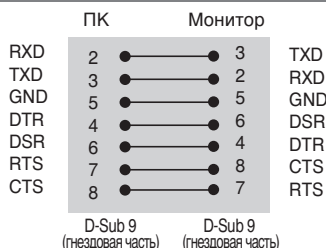
7-проводные конфигурации (стандартный кабель RS-232C)
