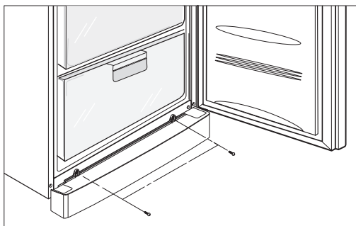
Рис 1. Установка нижней декоративной панели.
