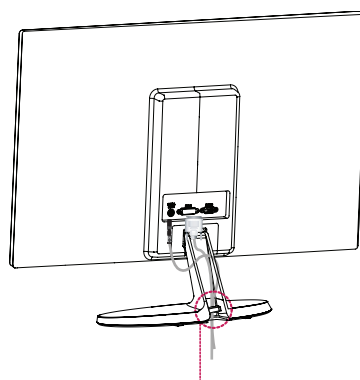
電纜支架
