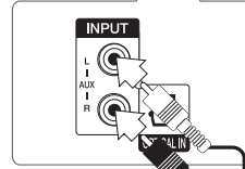
Ünitenin Arkası
