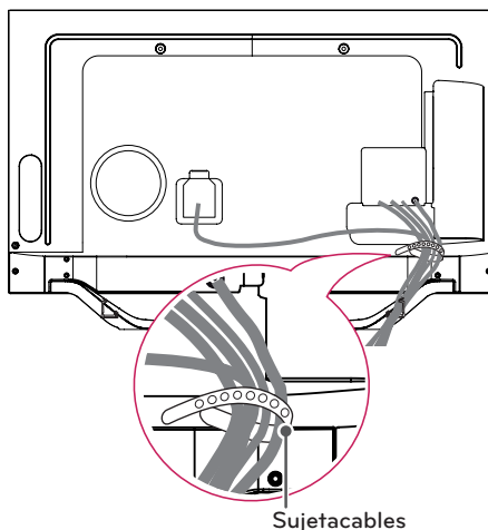
Sujetacables
