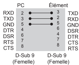
Configurations à 3 câbles (Non standard)
