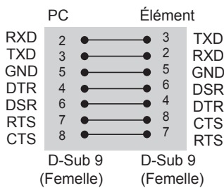
Configurations à 7 câbles (Câble standard RS-232C)
