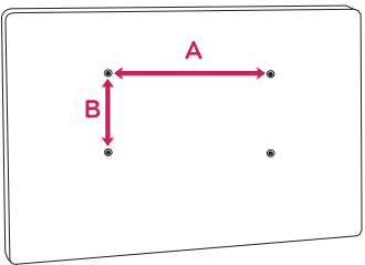
本体背面図
