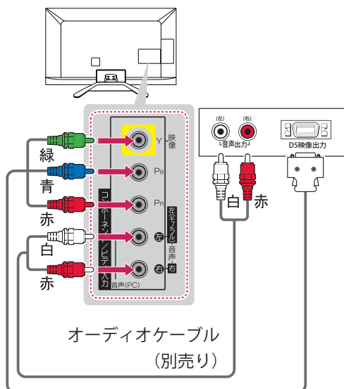
コンポーネント-D端子ケーブル (別売り)
