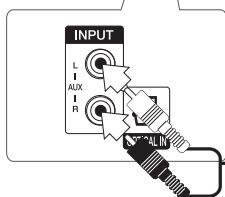
Iekārtas aizmugure
