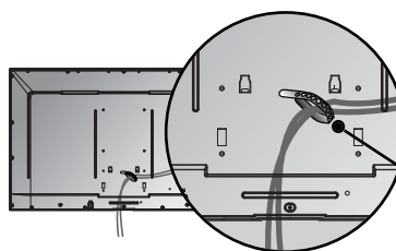
Uchwyt przewodów
