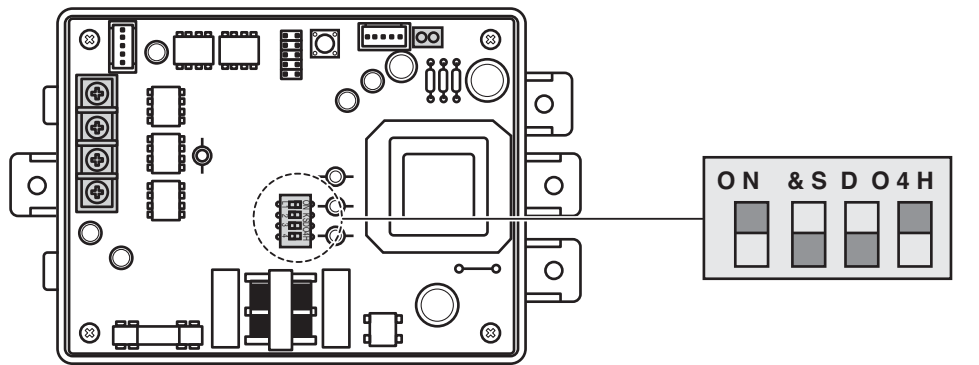
Impostazione dei microinterruttori
